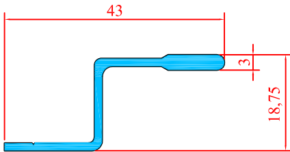
1922 0.287 Kg/m
