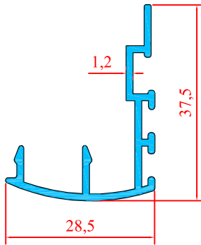
1902 0.318 Kg/m
