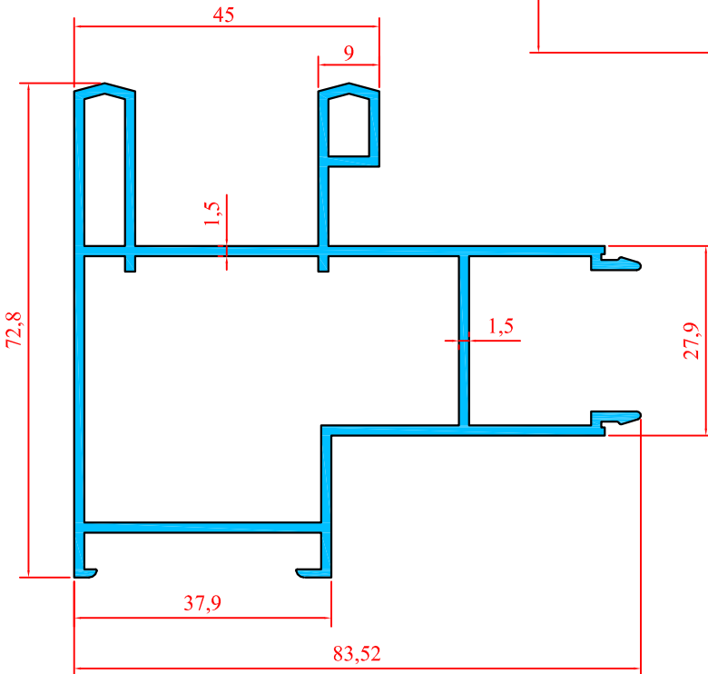
1913 1.512 Kg/m
