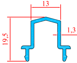
1920 0.194 Kg/m
