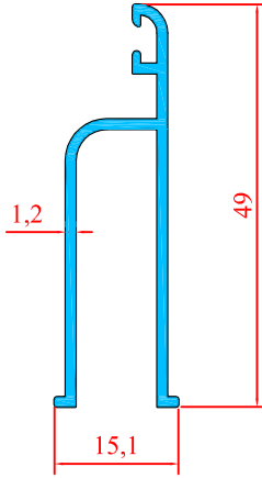
1916 0.331 Kg/m
