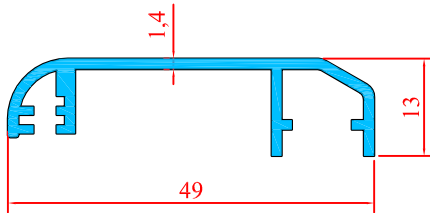
1918 0.355 Kg/m
