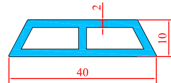
1230 0.489 Kg/m
