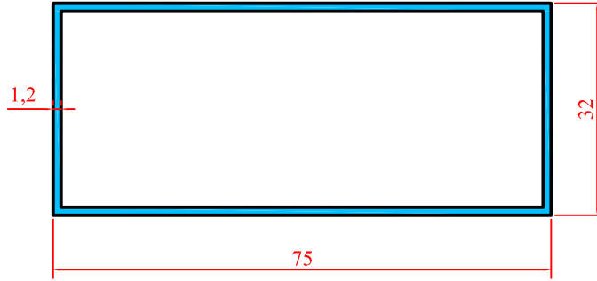
1001 0.683 Kg/m
