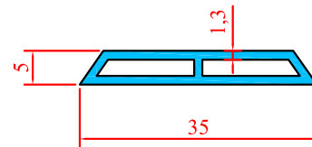
3665 0.251 Kg/m
